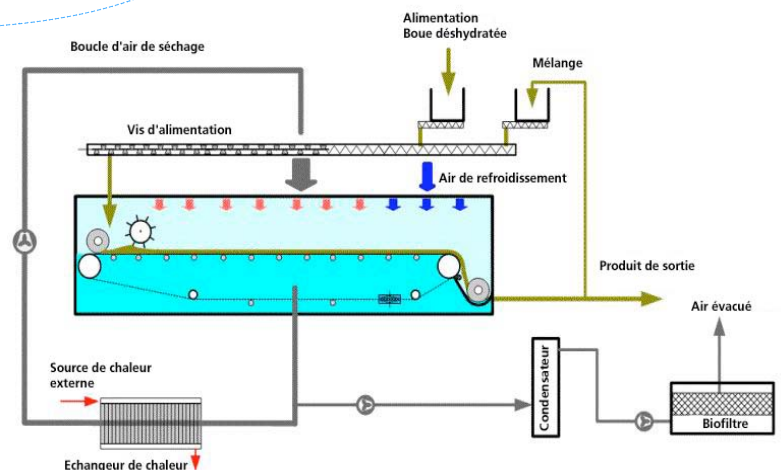
Le schéma ci-après représente un procédé de type « sécheur à bande »
