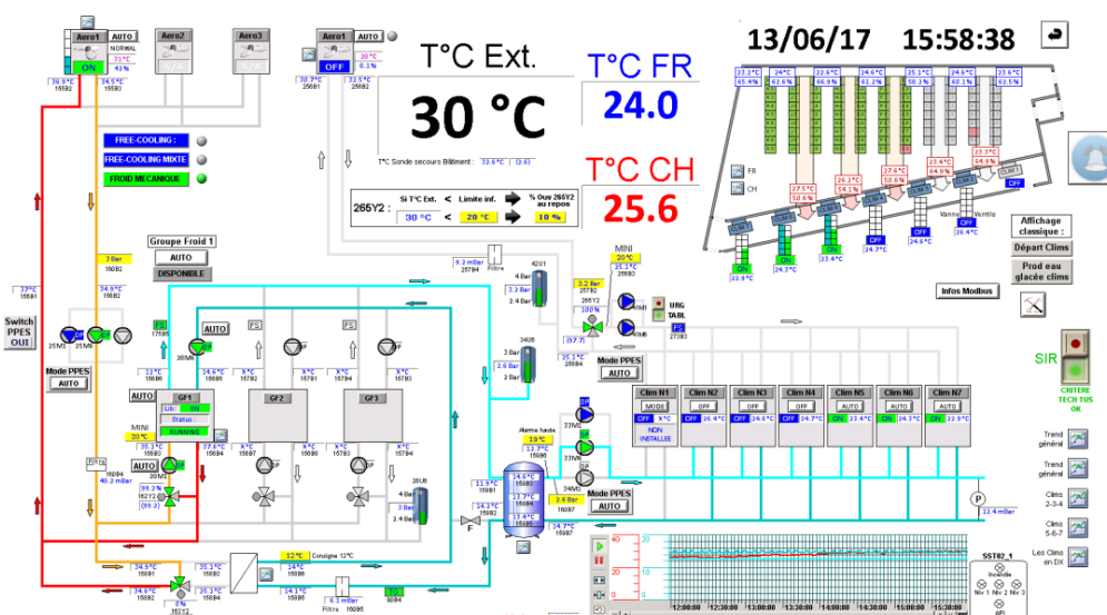
Schéma de principe d'installations techniques
