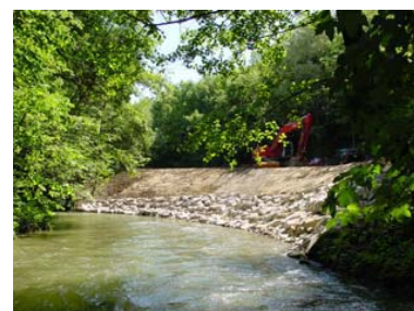
Situazione dopo i lavori, Réverule
