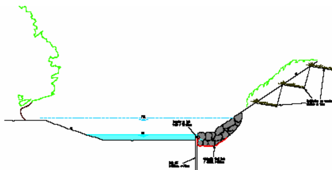
Sezione tipo progettata
