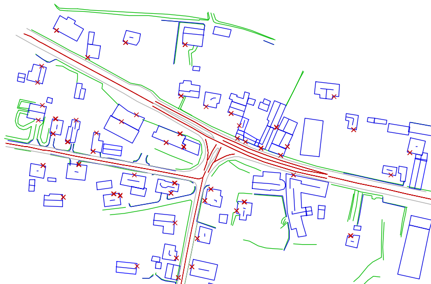
Planimetria SLIP di Coldrerio 1:2500 – Sorgenti e punti d'immissione
