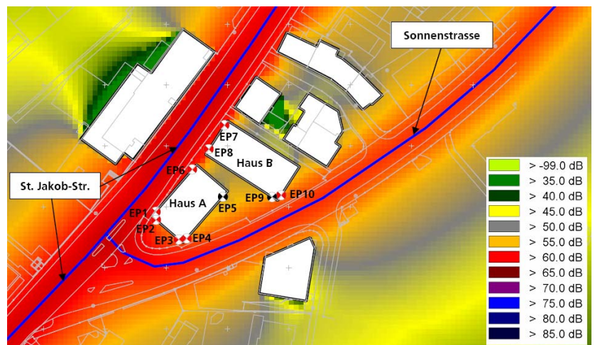
Lärmbelastungskarte mit Lage der geplanten Gebäude und Empfangspunkte (EP) sowie der Lärmquellen (Strassen)
