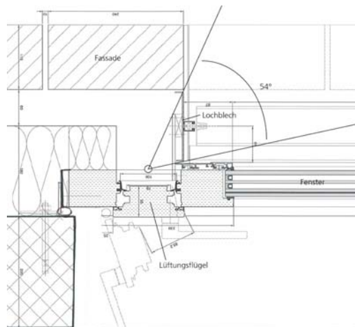
Spezielle Lüftungseinrichtung
